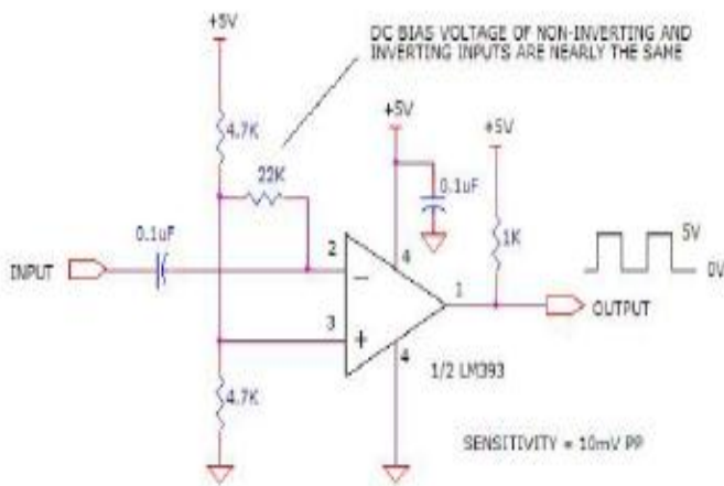
Fig. 7. ZCD circuit
